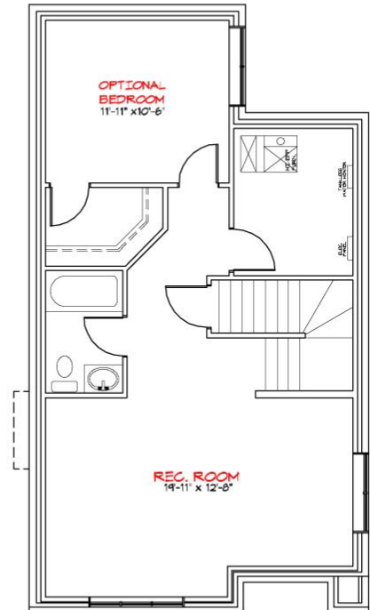
OPTIONAL BASEMENT LAYOUT
